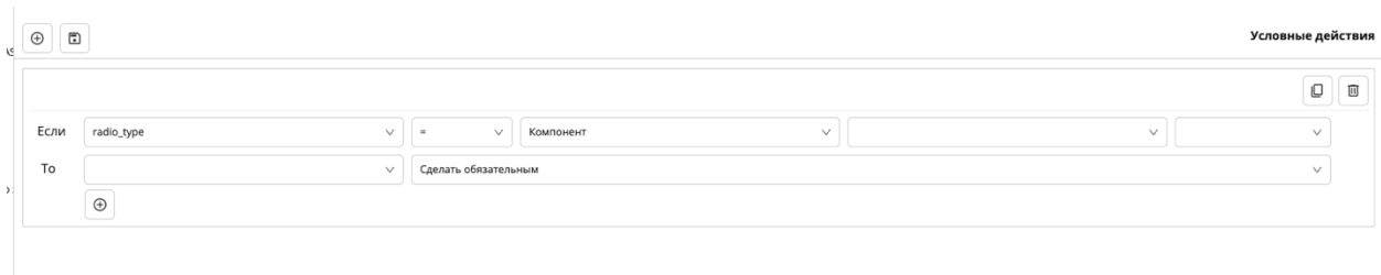
Рис. 18: Настройка условия
