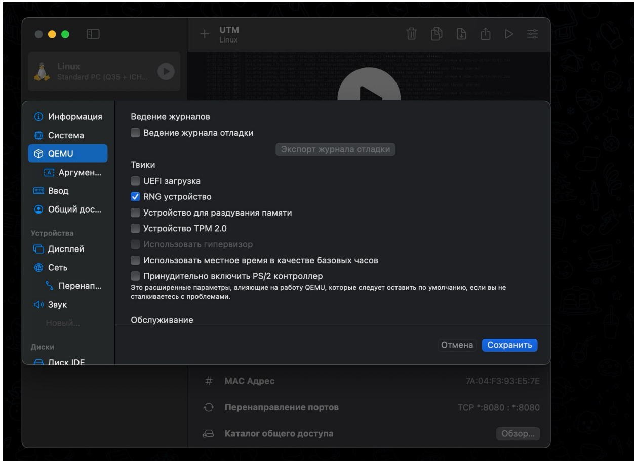
Рис. 9: Настройки QEMU
