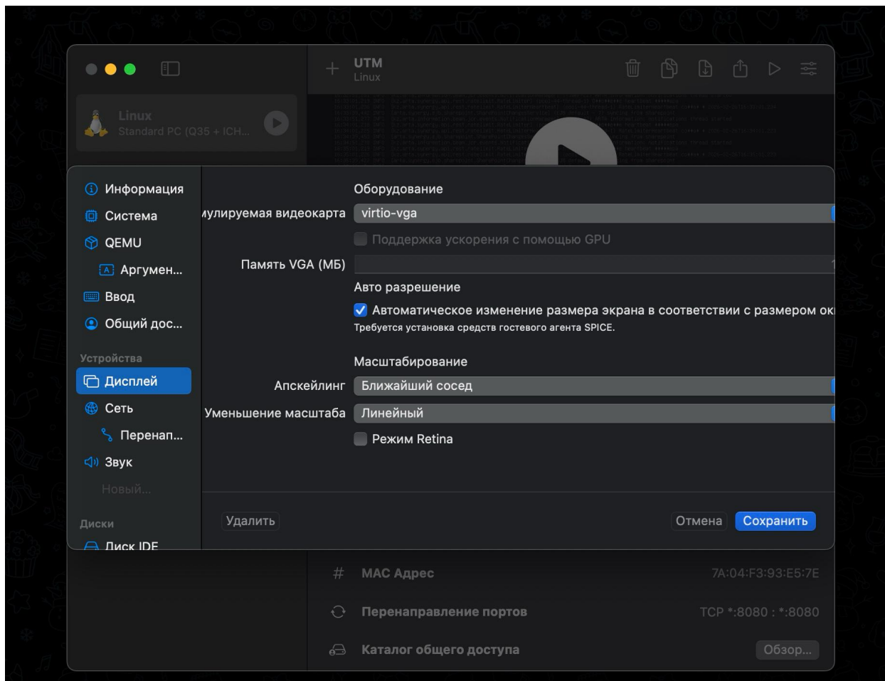
Рис. 10: Настройки дисплея
