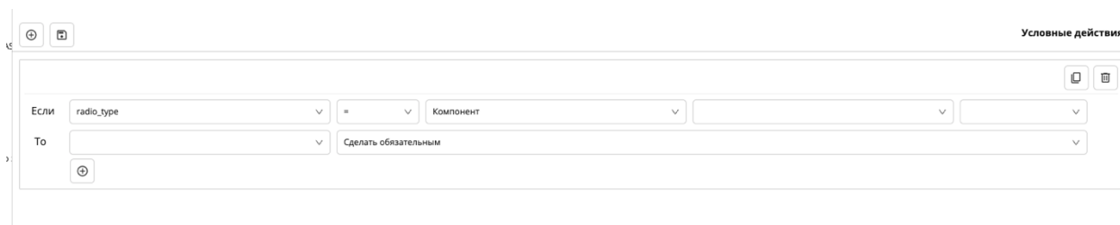
Рис. 18: Настройка условия
