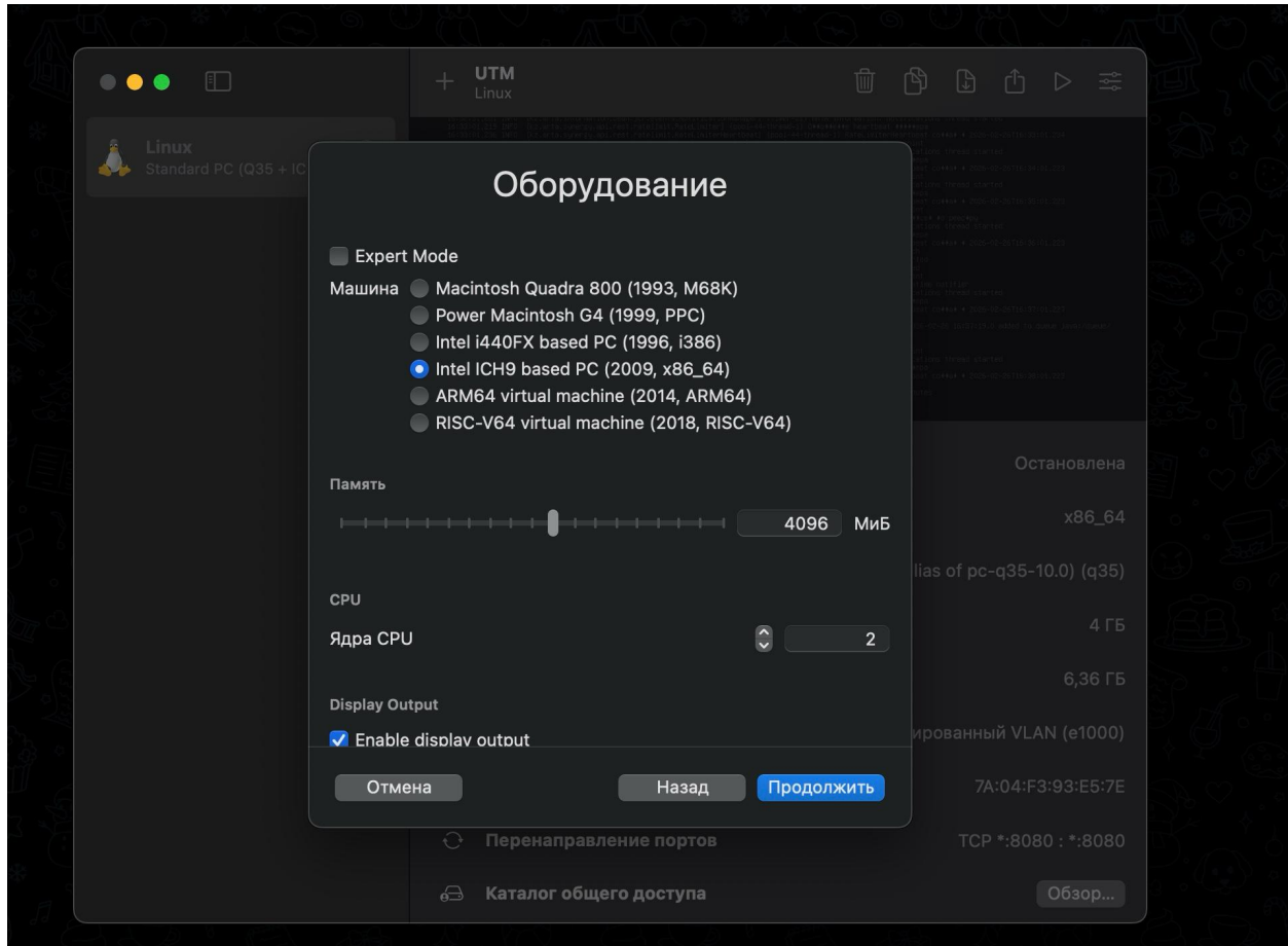
Рис. 6: Настройка ресурсов
