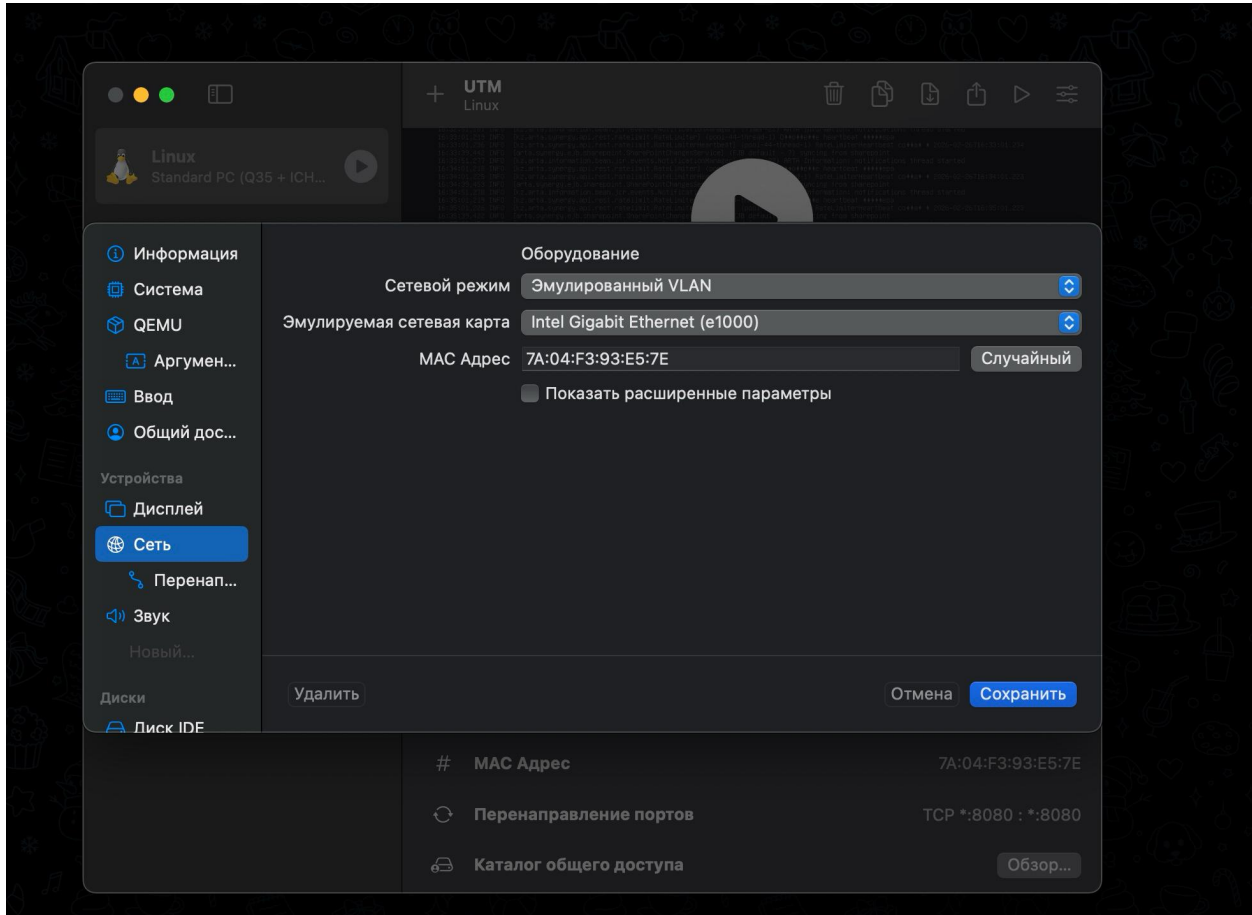
Рис. 11: Настройка сети
