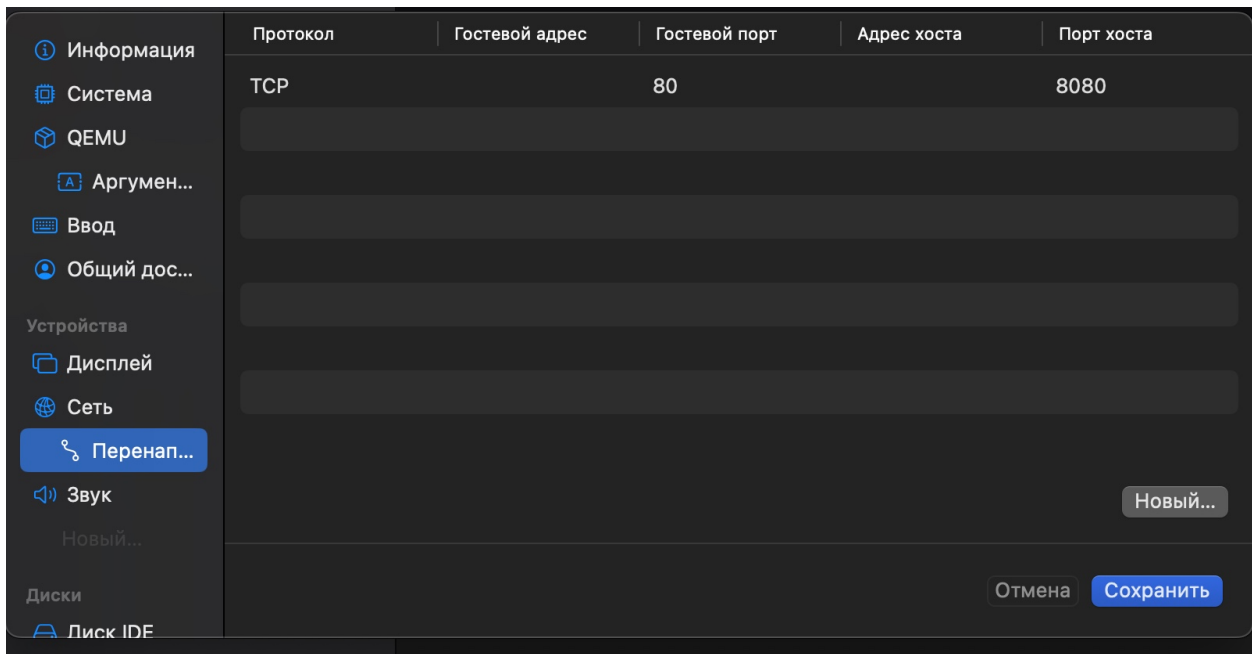
Рис. 12: Проброс портов
