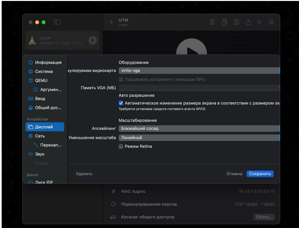
Рис. 10: Настройки дисплея
