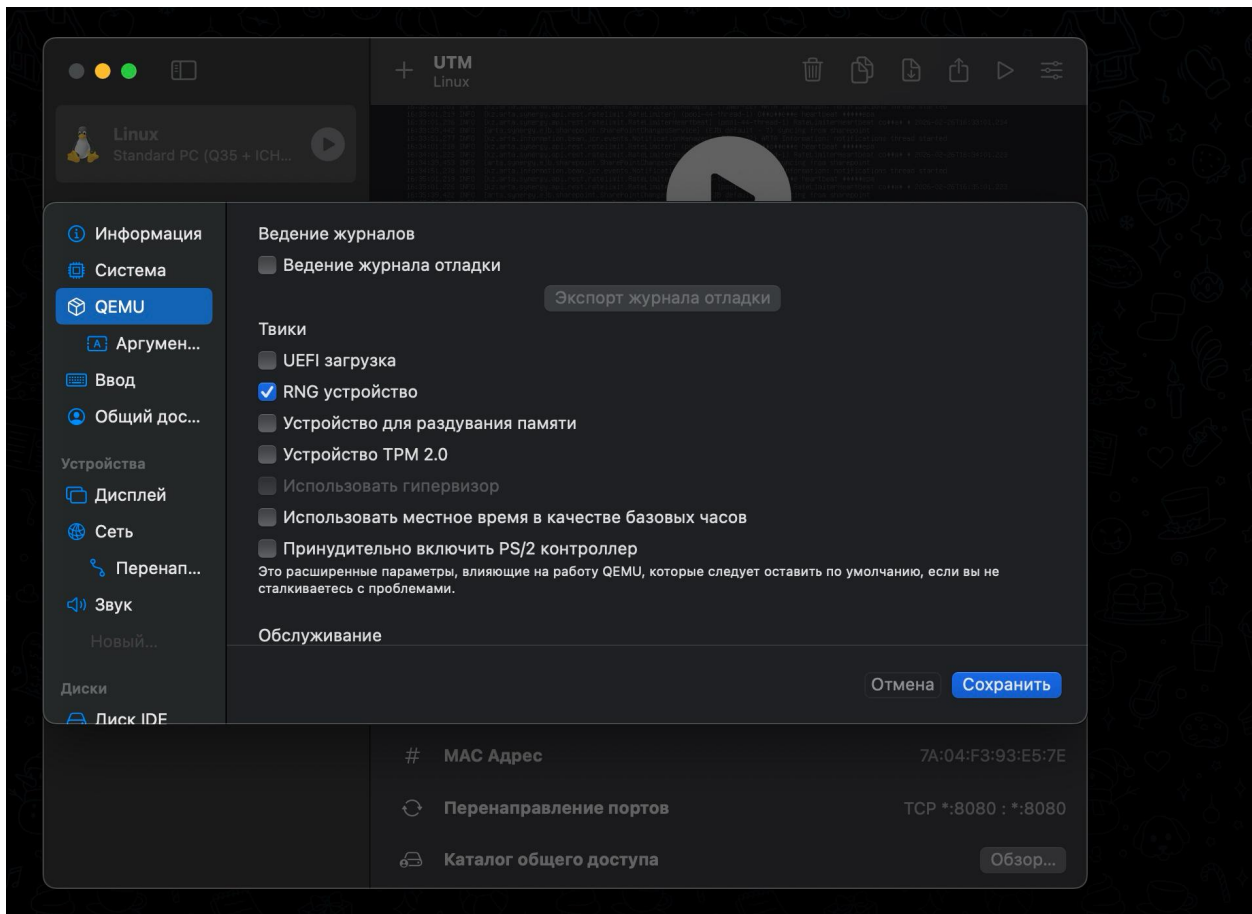
Рис. 9: Настройки QEMU
