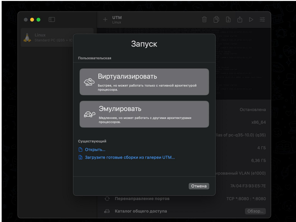
Рис. 4: Режим эмуляции
