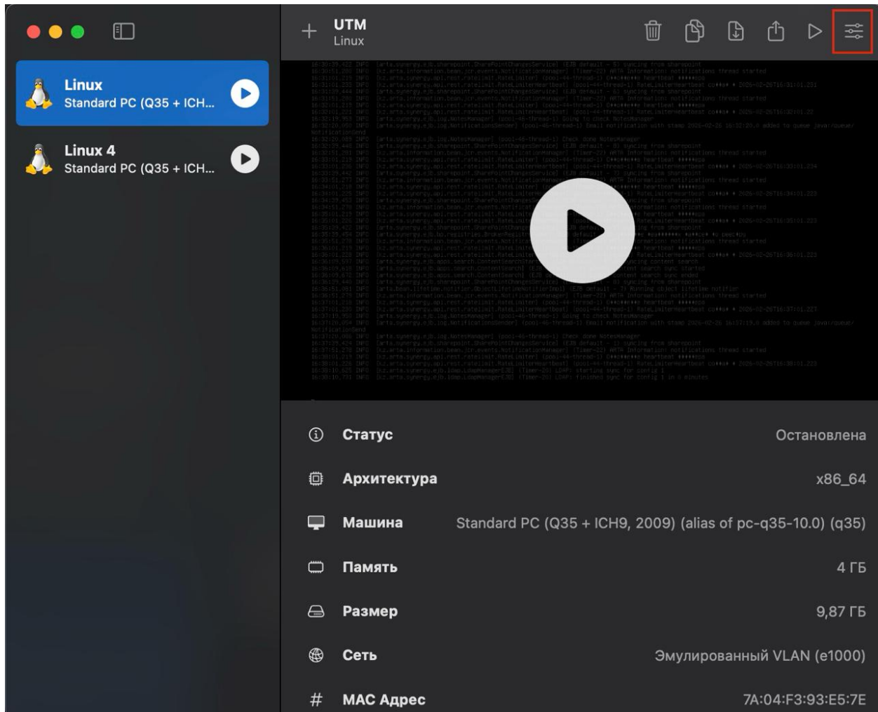
Рис. 8: Дополнительные настройки
