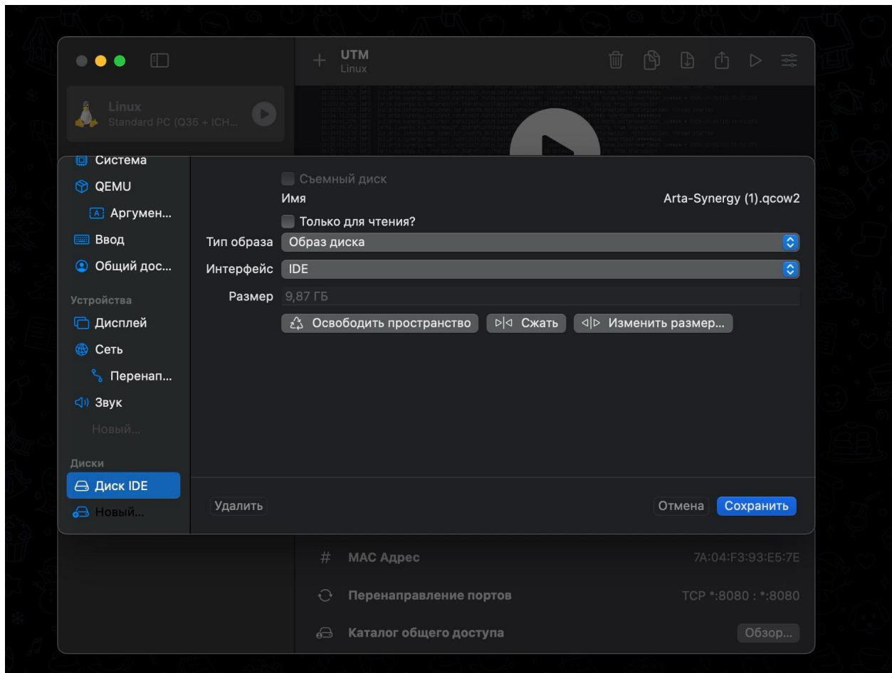
Рис. 13: Настройки диска
