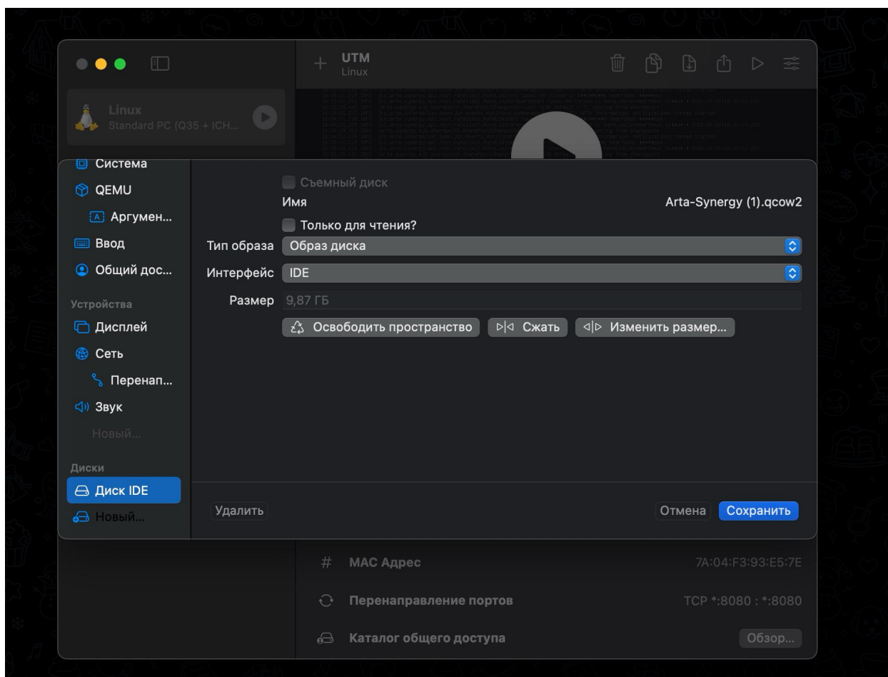
Рис. 13: Настройки диска
