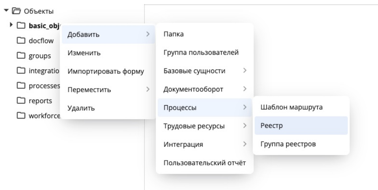
Рис. 1: Создание реестра
