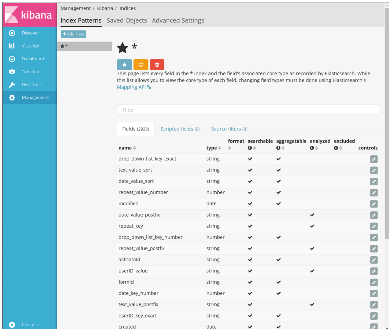
Рис. 3: Созданный шаблон индексов
