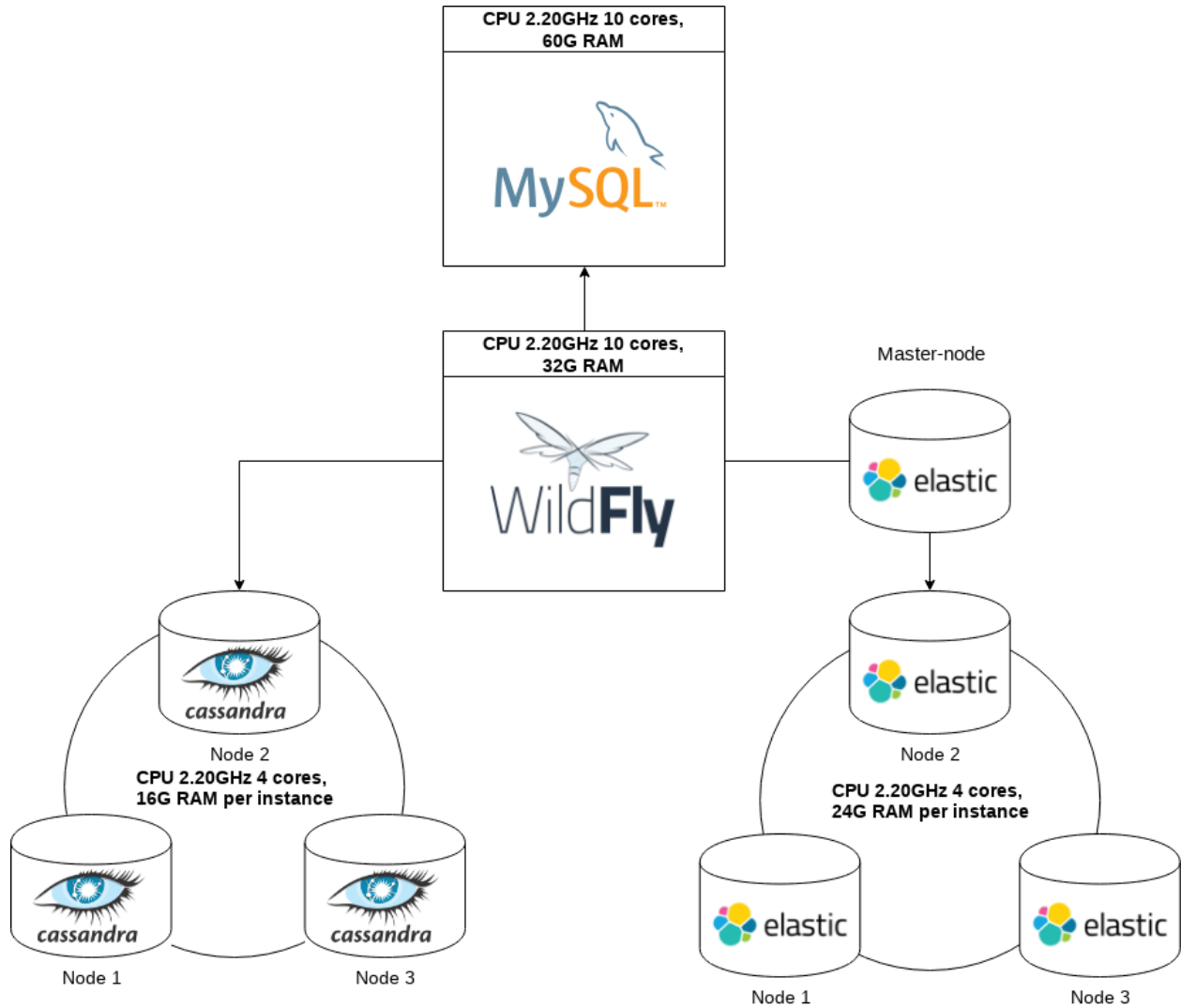
Рис. 4: Схема инфраструктуры платформы для production mode
