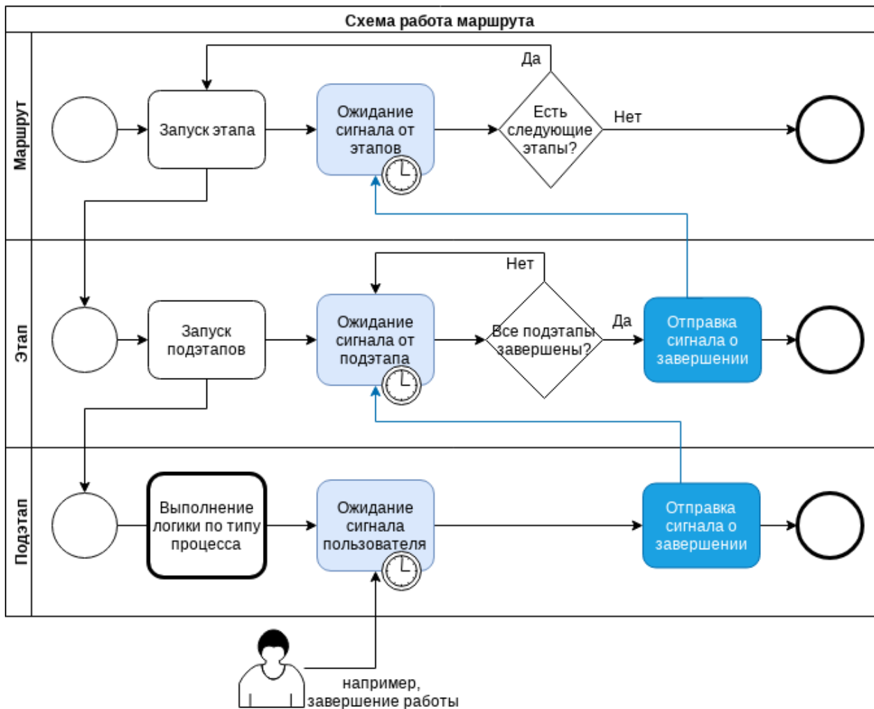
Рис. 6: Логика выполнения маршрута
