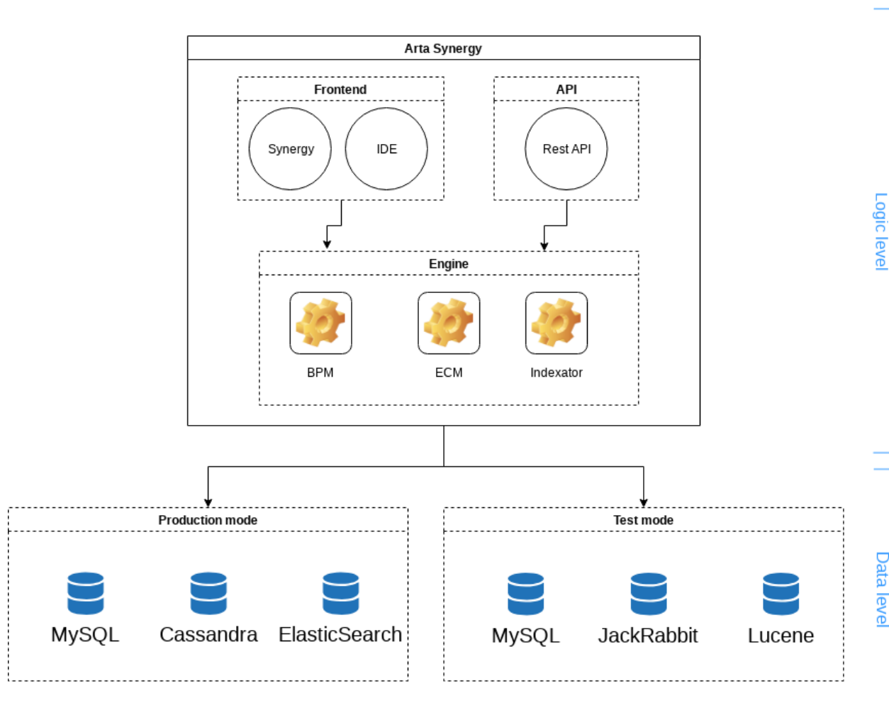
Рис. 3: Верхнеуровневая архитектура платформы
