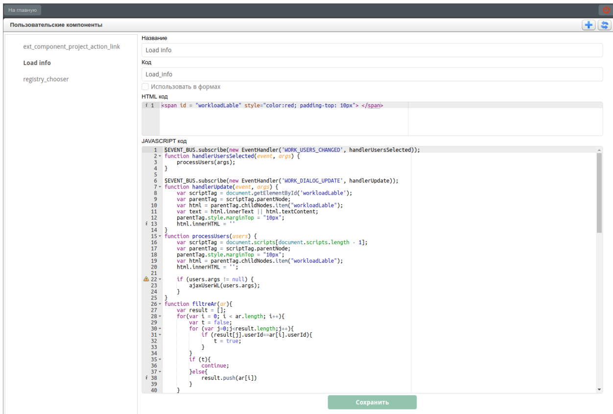
Рис. 1: Пользовательские компоненты
