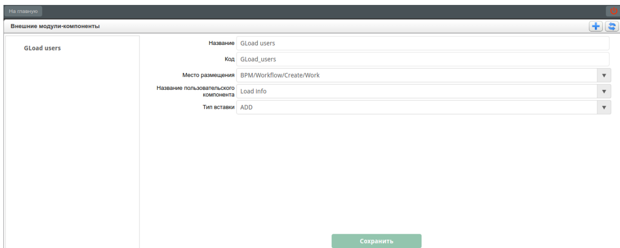
Рис. 2: Внешние модули-компоненты
