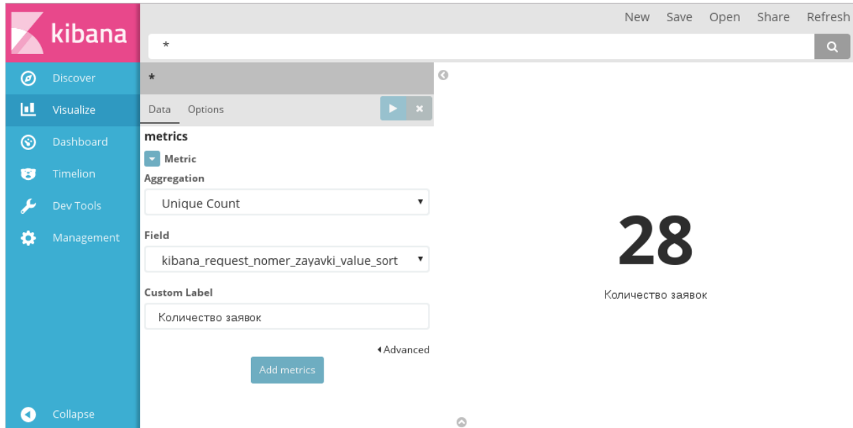
Рис. 22: Создание Metrics
