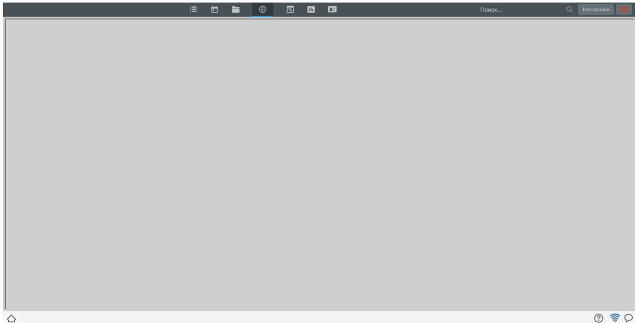
Рис. 2: Внешний WEB-модуль
